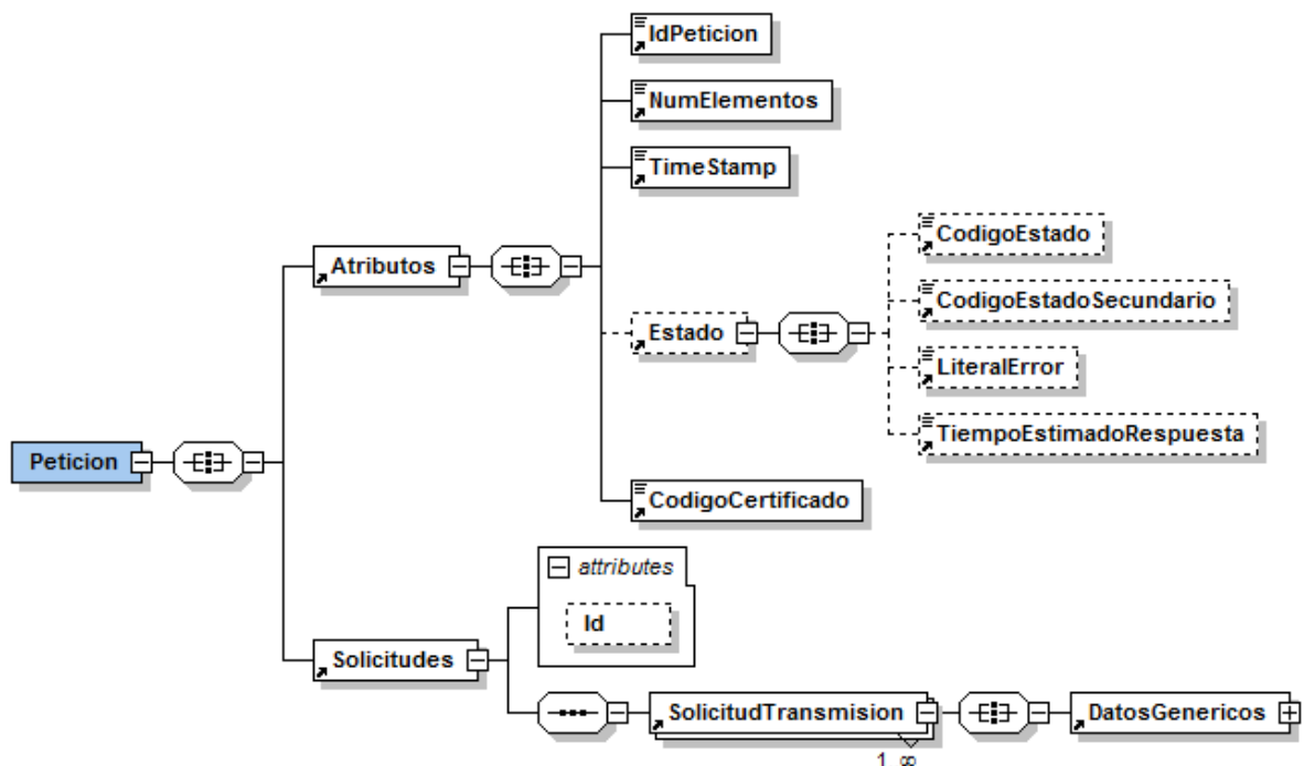
Figura 5.- Mensaje de petición al Servicio de Consulta de Matrimonio
