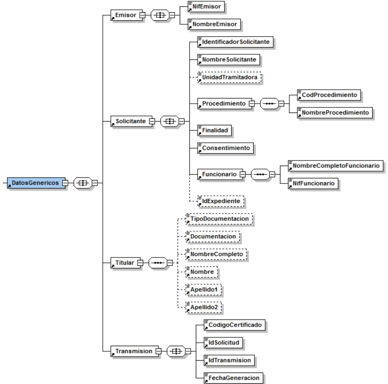
Figura 8.- Contenido del Nodo DatosGenericos del Servicio de Consulta de Matrimonio
