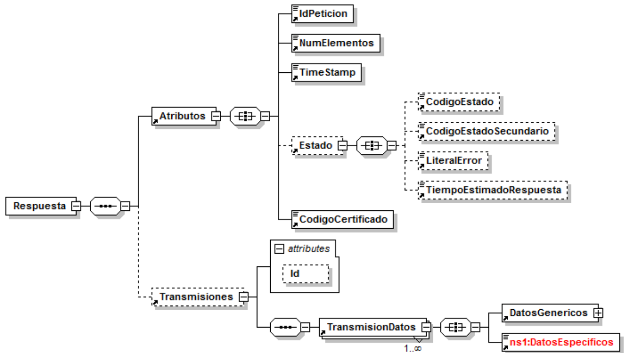
Figura 7.- Mensaje de respuesta del Servicio de Consulta de Matrimonio
