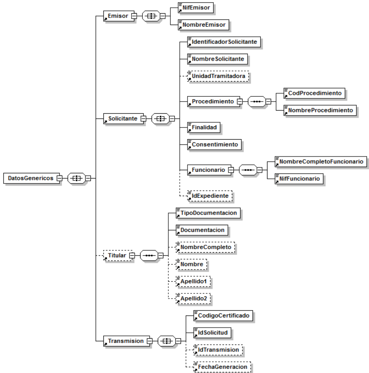
Figura 6. Diagrama de la rama de DatosGenericos del mensaje de petición del Servicio
