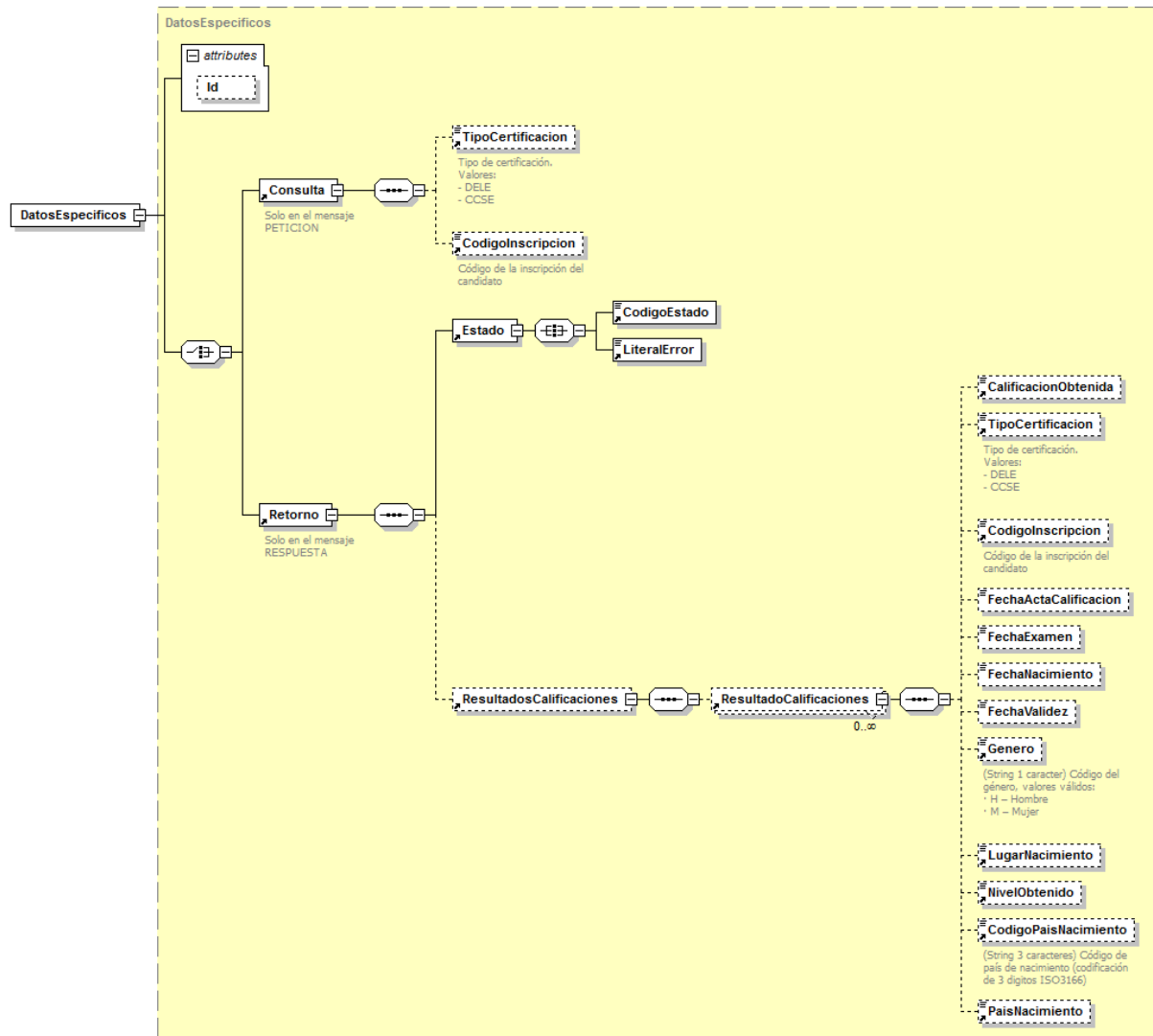
Figura 9. Diagrama de Datos Específicos de Respuesta del Servicio
